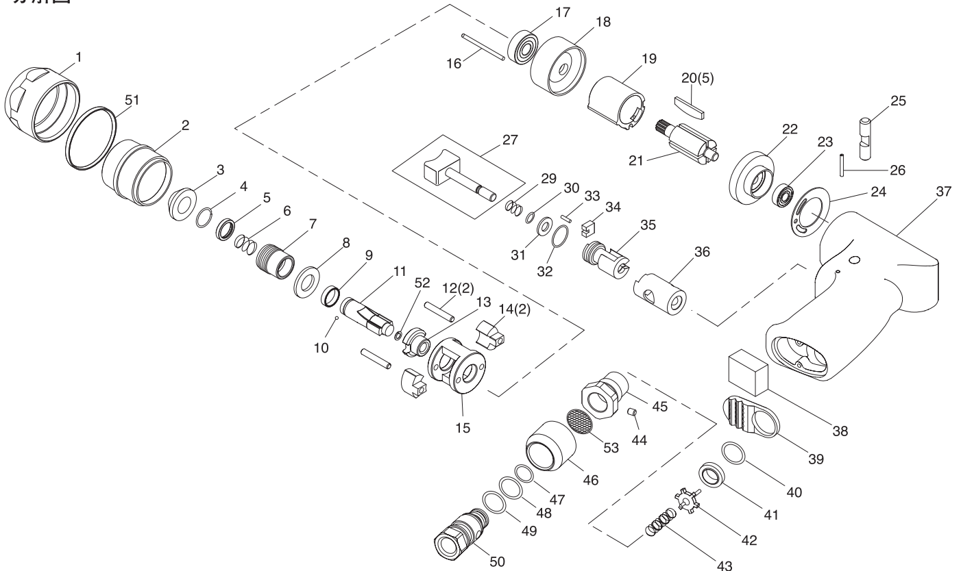
分解図
