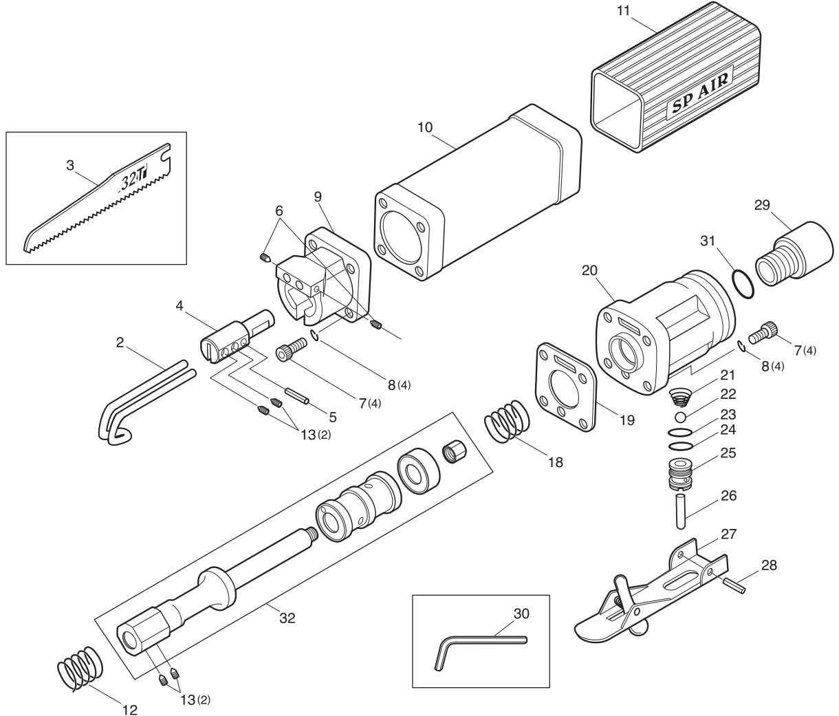
分解図
