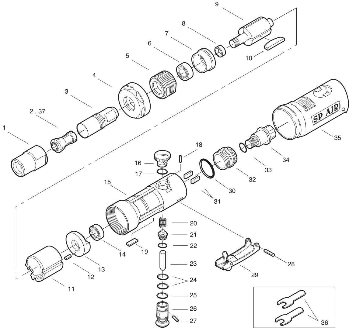
分解図
