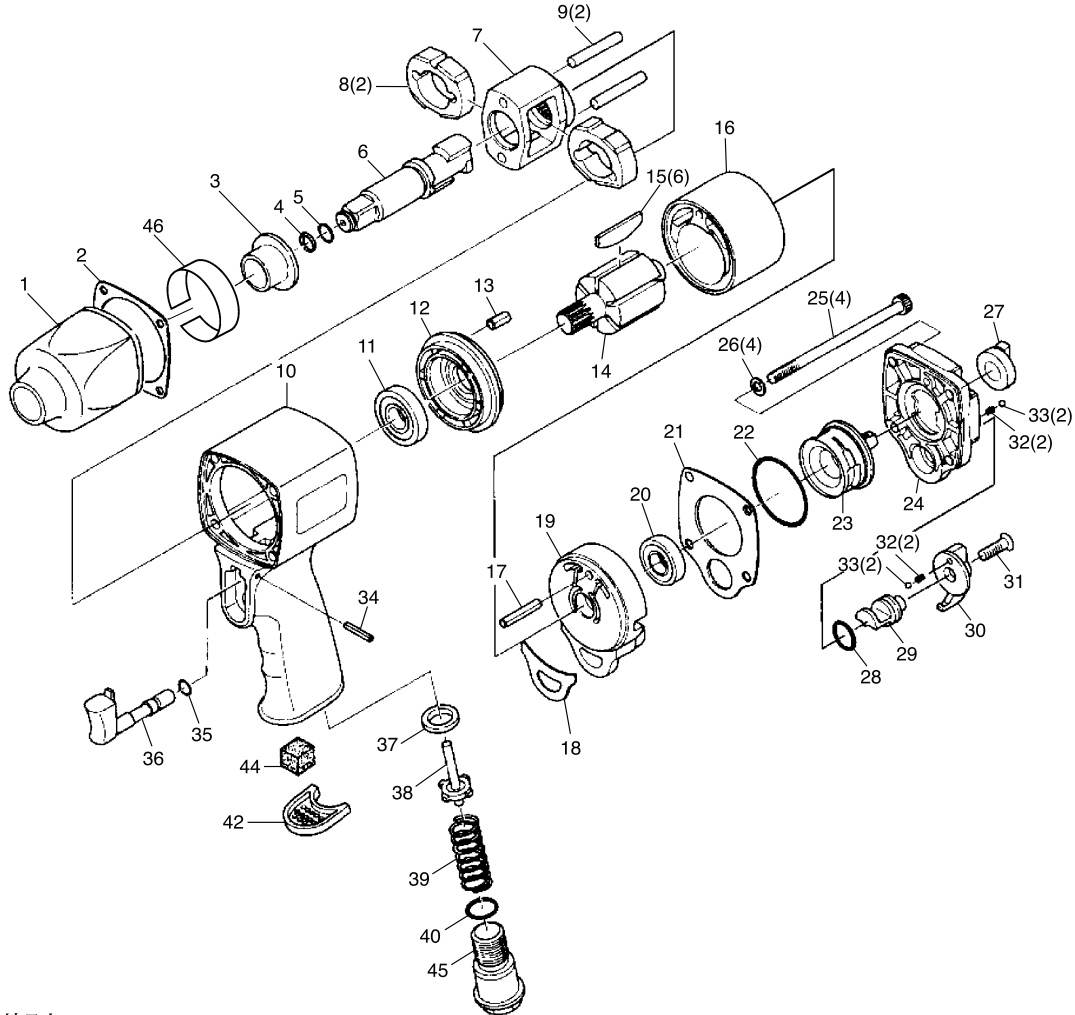
分解図
