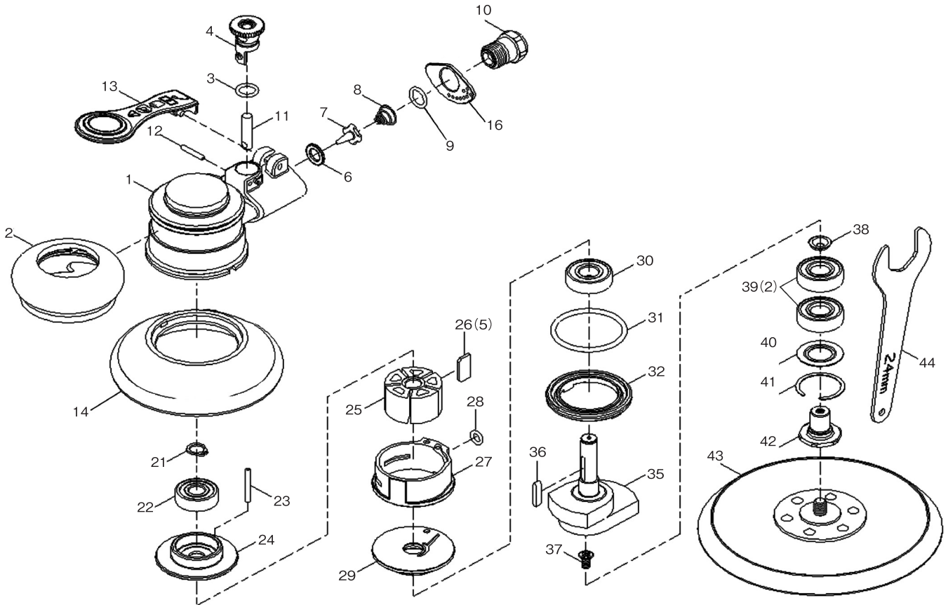
分解図
