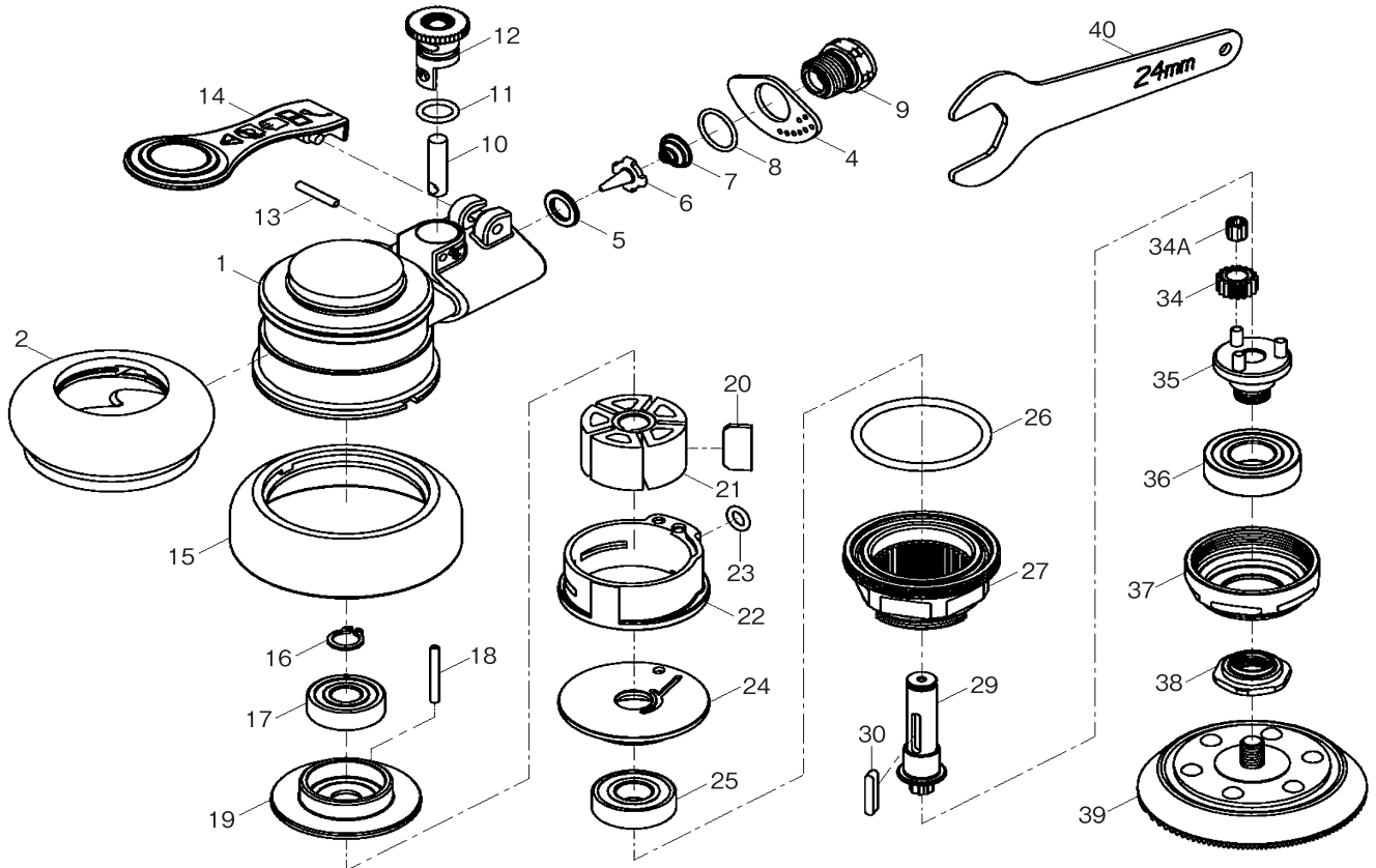
分解図
