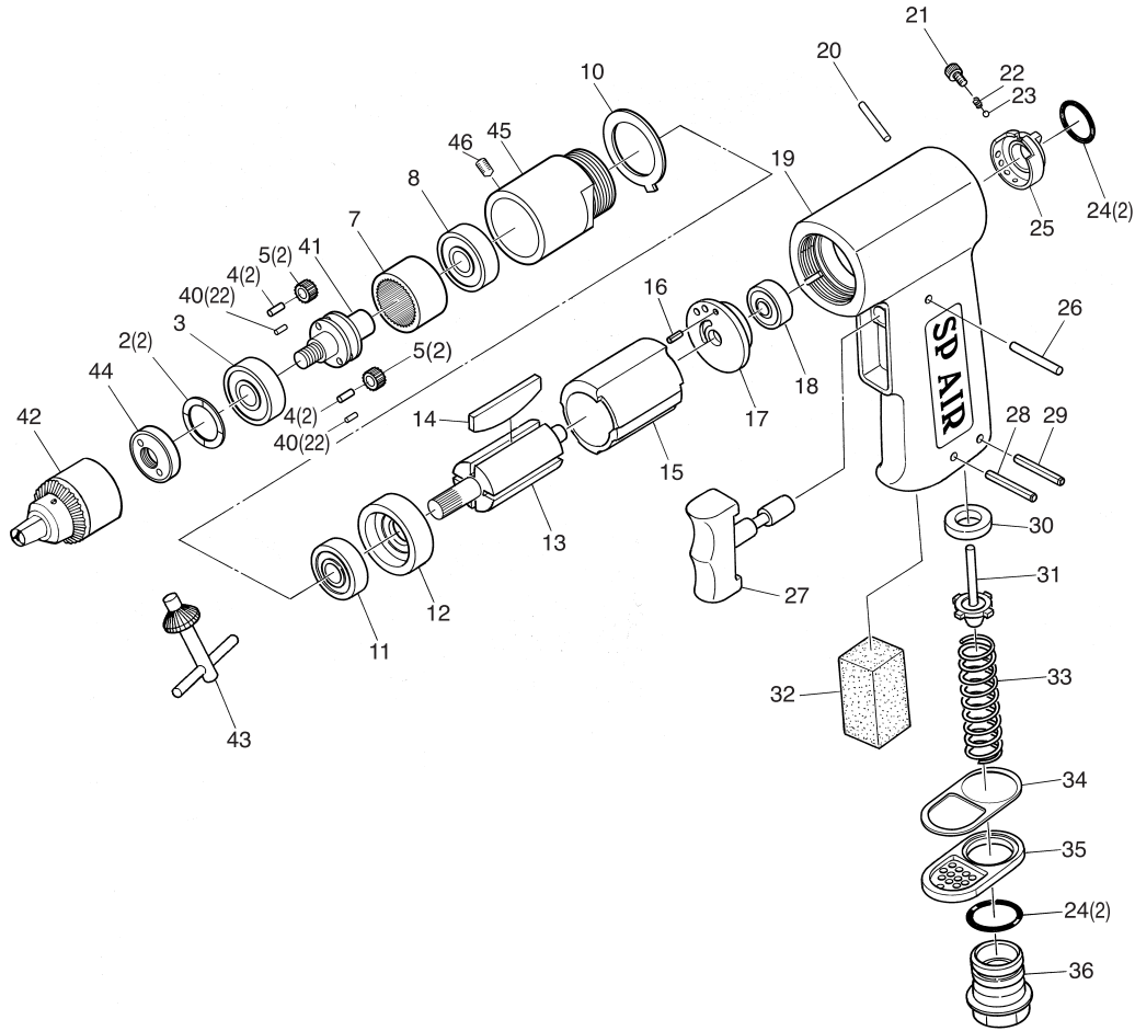
分解図
