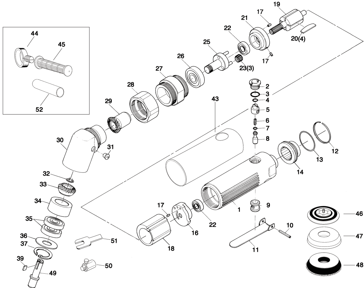
分解図
