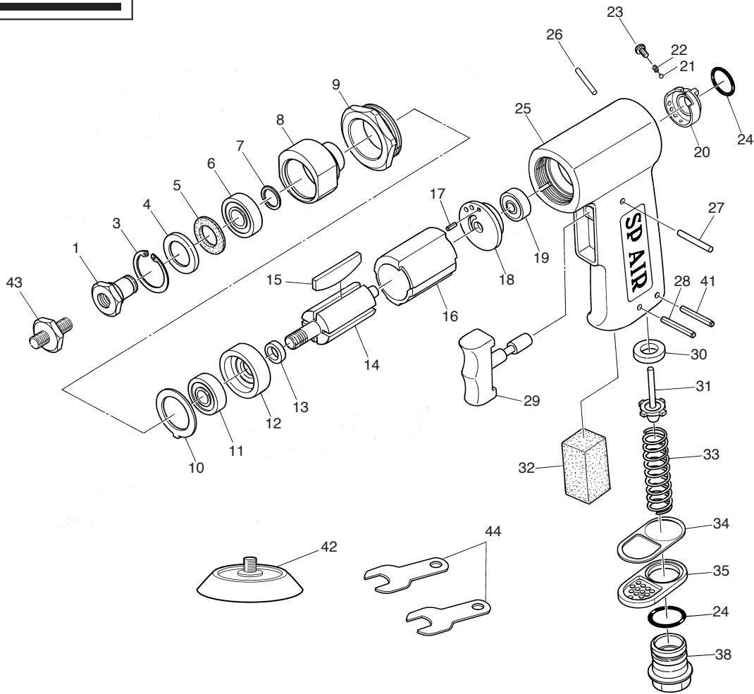
パーツプライスリスト
